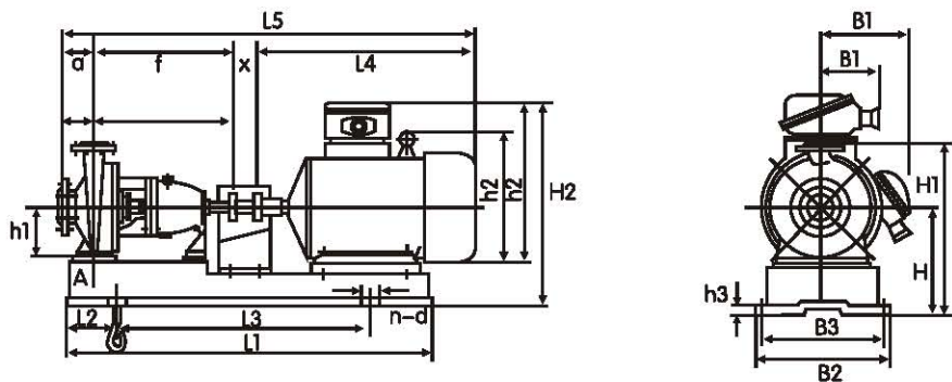
图5 IH化工泵外型尺寸图
