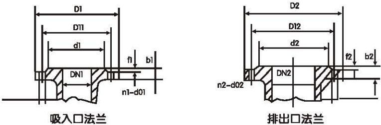
图 4 IH型化工泵进出口法兰示意图
