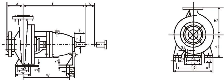
图 3 IH型化工泵外型尺寸图
